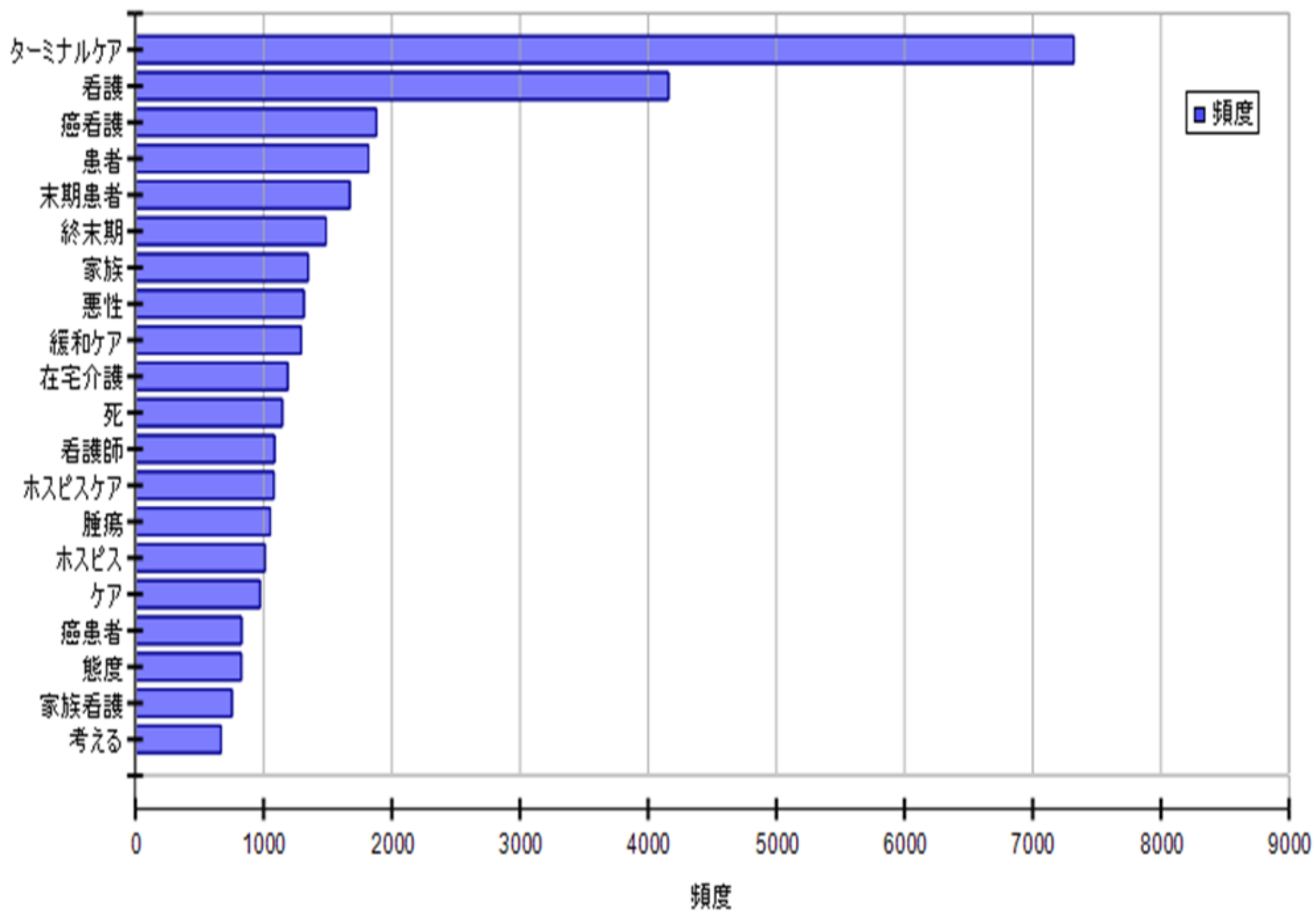
図2 単語頻度
