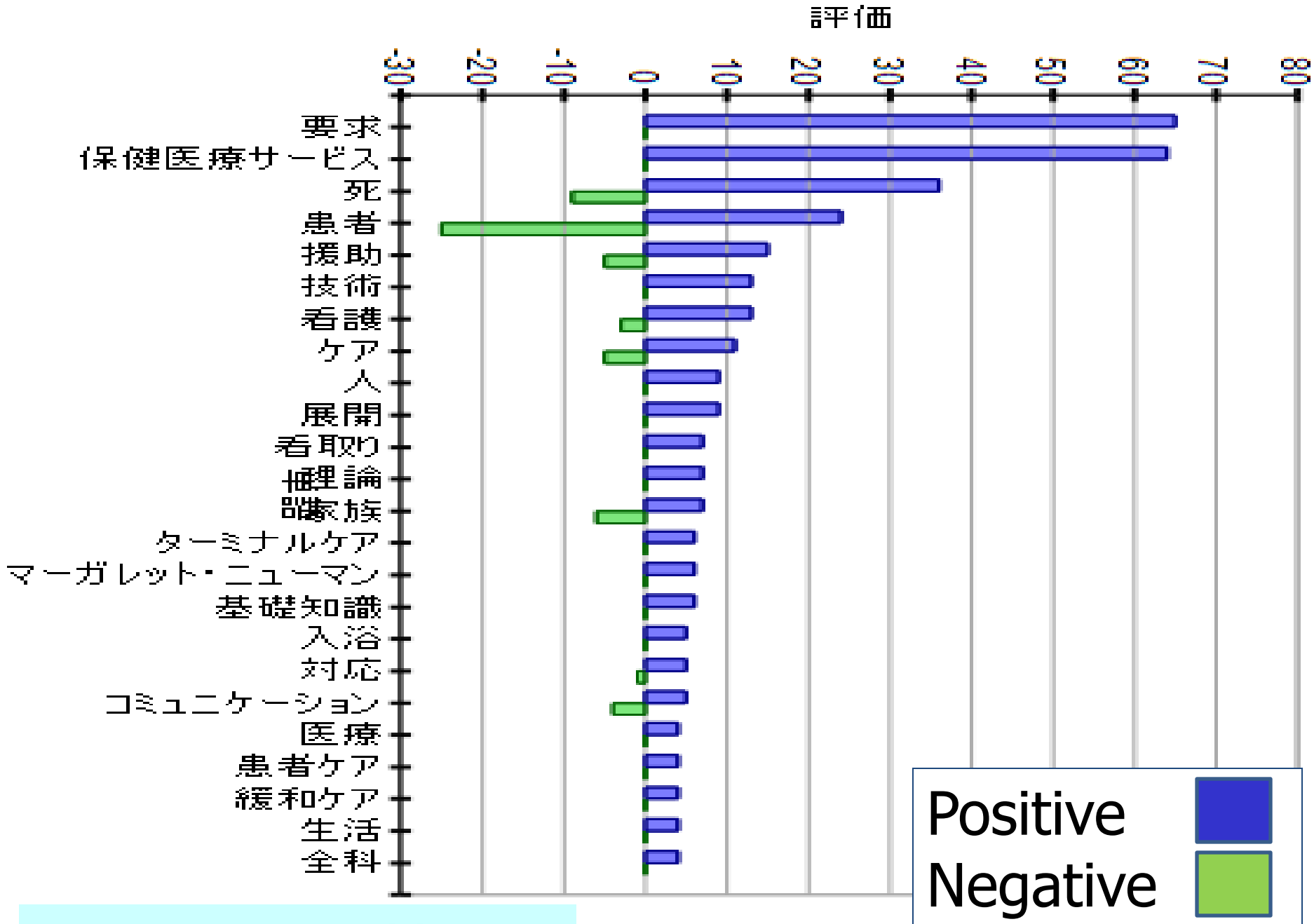
図4 評判抽出
